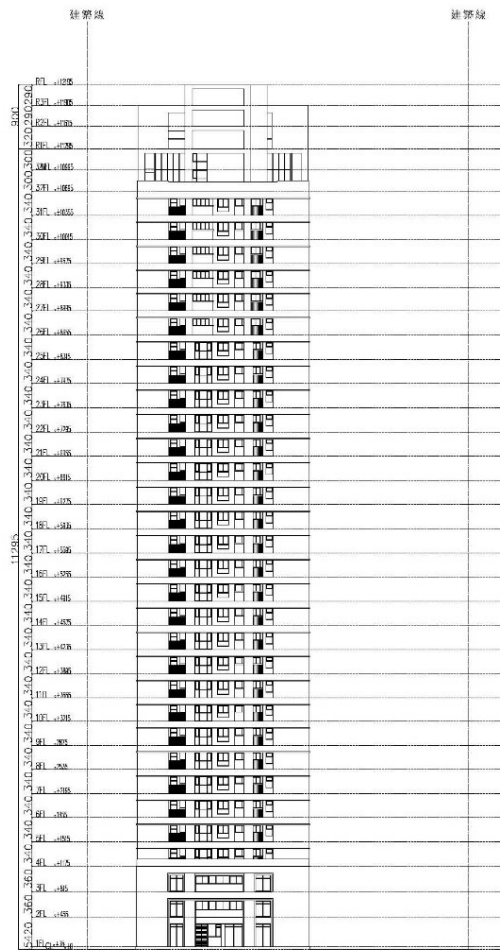
A、B棟右側立面圖 S:1/600
