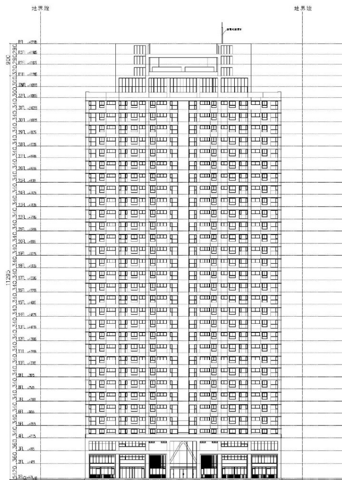
A、B棟背向立面圖 S:1/600
