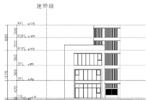
C棟右側立面圖 S:1/300
